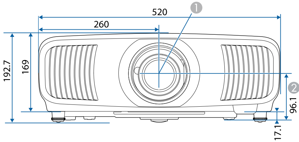
1 Centre de l'objectif (lorsque l'objectif est au centre)
