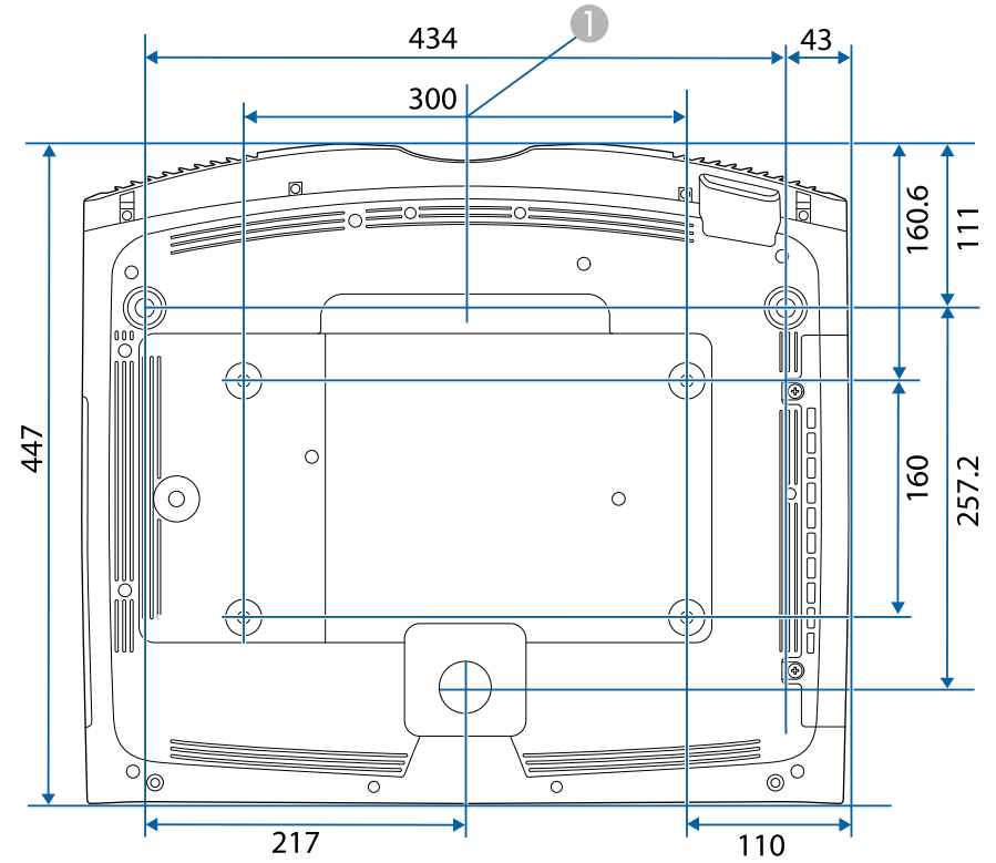
2 Distance entre le centre de l'objectif et le trou de montage pour bride de suspension
